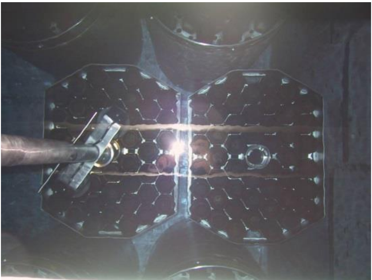
Obr. č. 12: Zásobníky s VJP
