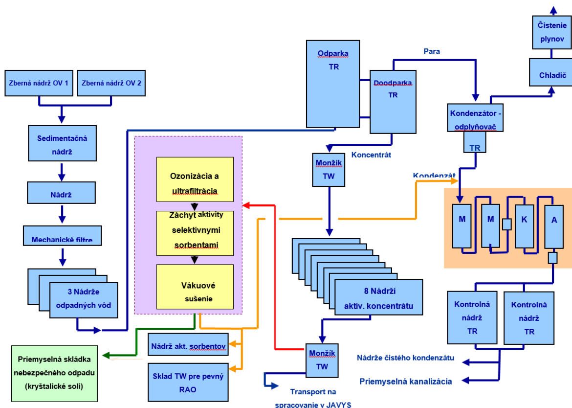
Obr. č. 28 Schéma spracovania rádioaktívnych kvapalných koncentrátov v JE Mochovce
