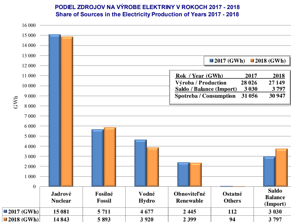
Obr. č. 2 Podiel zdrojov na výrobe elektriny v rokoch 2017 – 2018 (zdroj: SEPS, a. s.)
