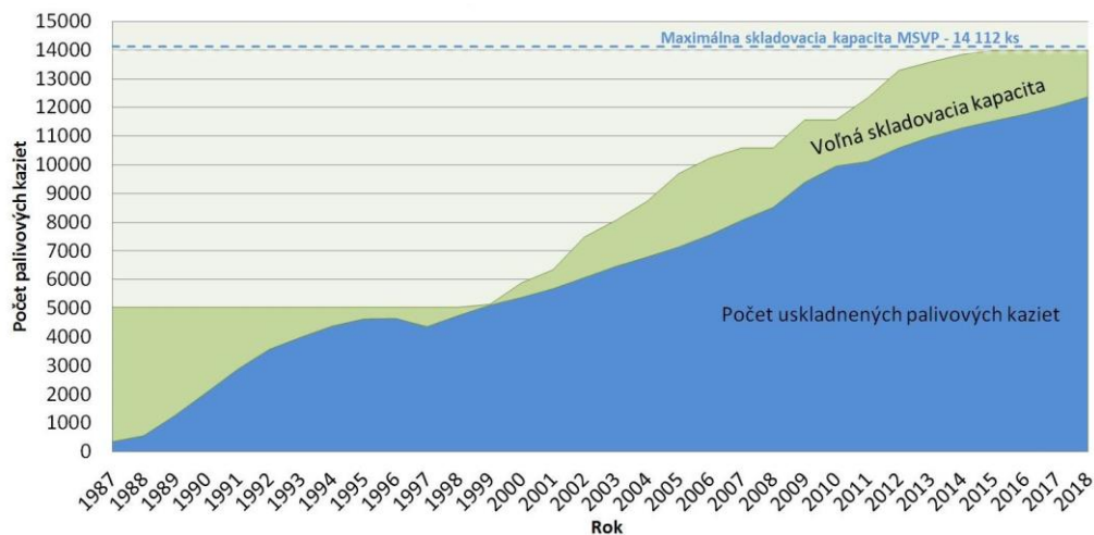
Obr. č. 9 Priebeh postupného zaplňania MSVP vyhoretým jadrovým palivom k 31.12.2018
