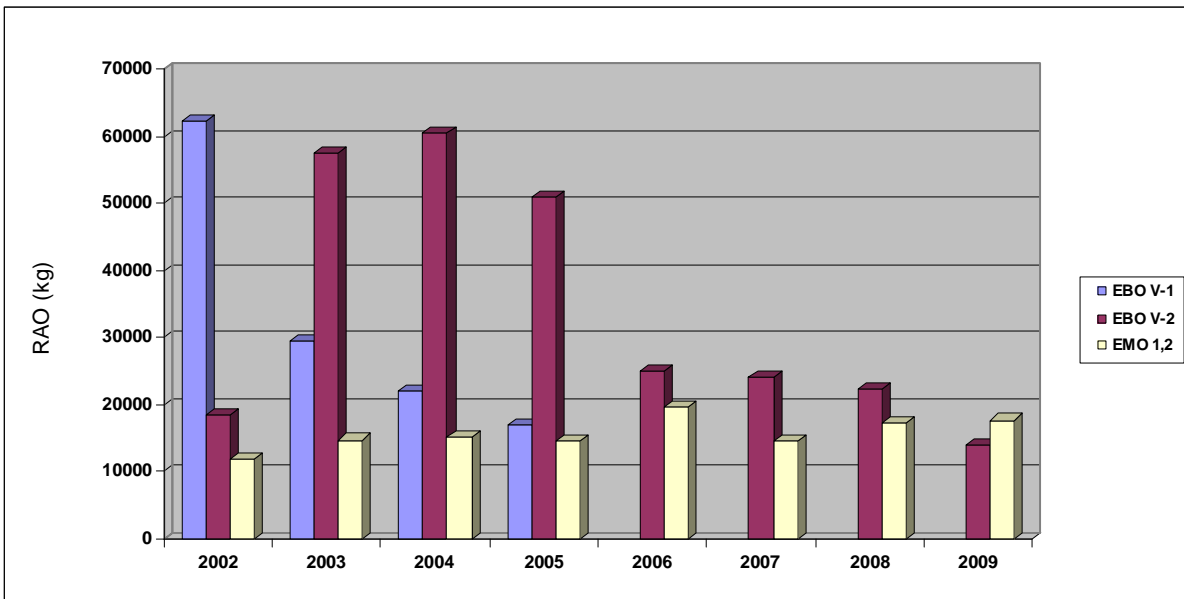
obr.5.3.6 Tvorba pevných RAO v SE-EBO, EMO pre EBO V-1
