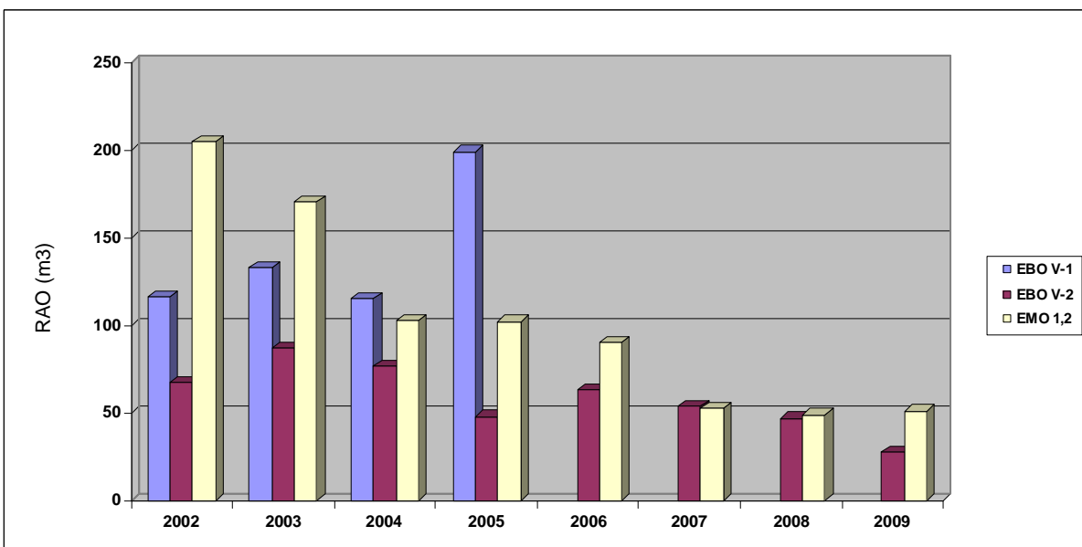
obr.5.3.7 Tvorba kvapalných RAO v SE-EBO, EMO pre EBO V-1
